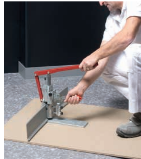
Outil de découpe «grugeoir» recommandé.
